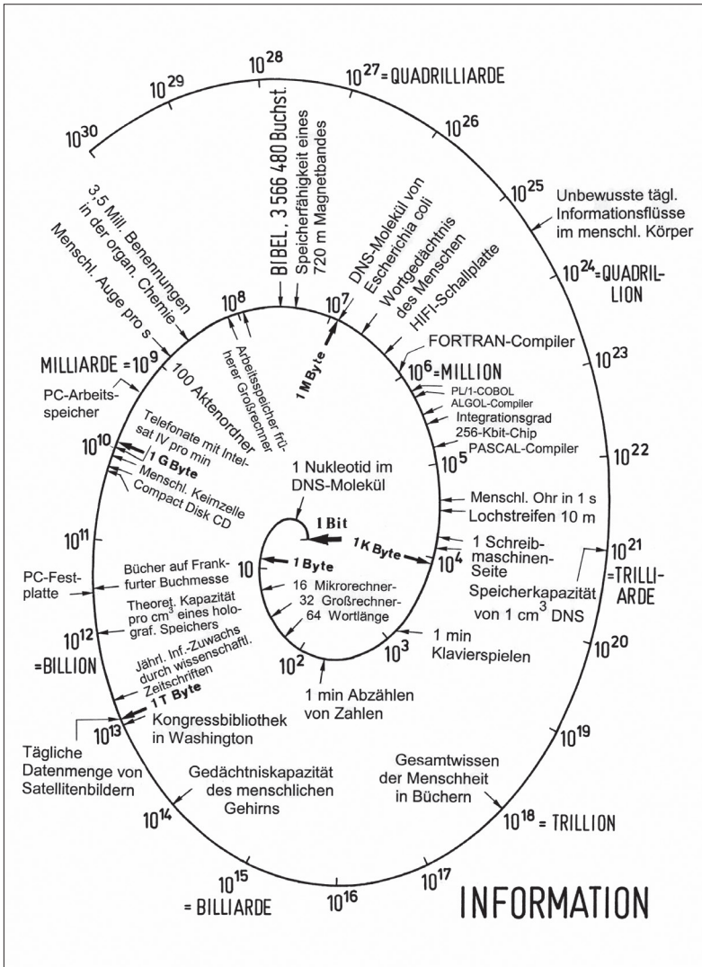
Bild 39: Die Informationsspirale
